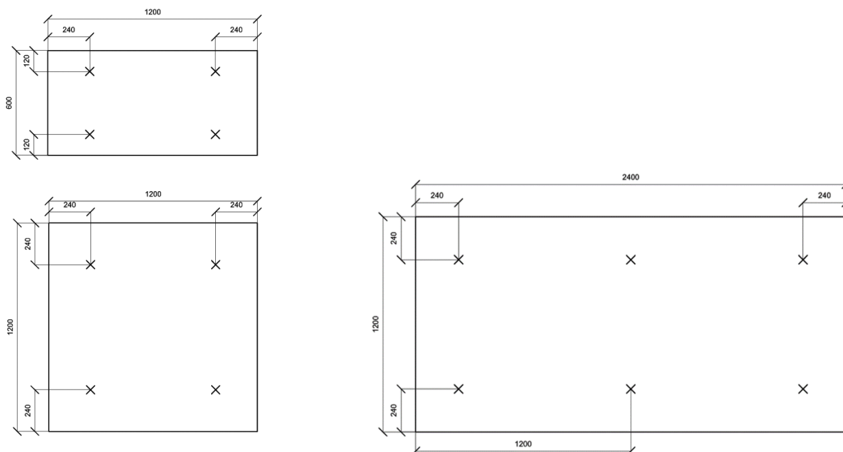
Fig. 1 – Plaatsingspatronen voor de mechanische bevestigingen
